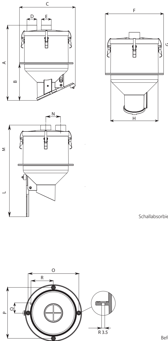
Draufsicht, Positionierschablone
