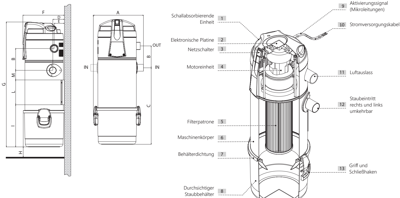
Schnittzeichnung ENVIRON LOADER 900
