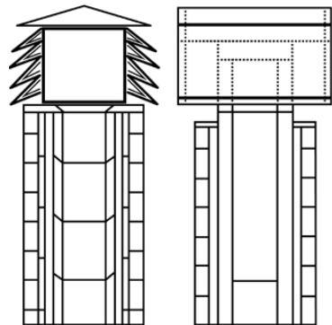
SCHORNSTEINAUSGANG (WINDSCHUTZ)
